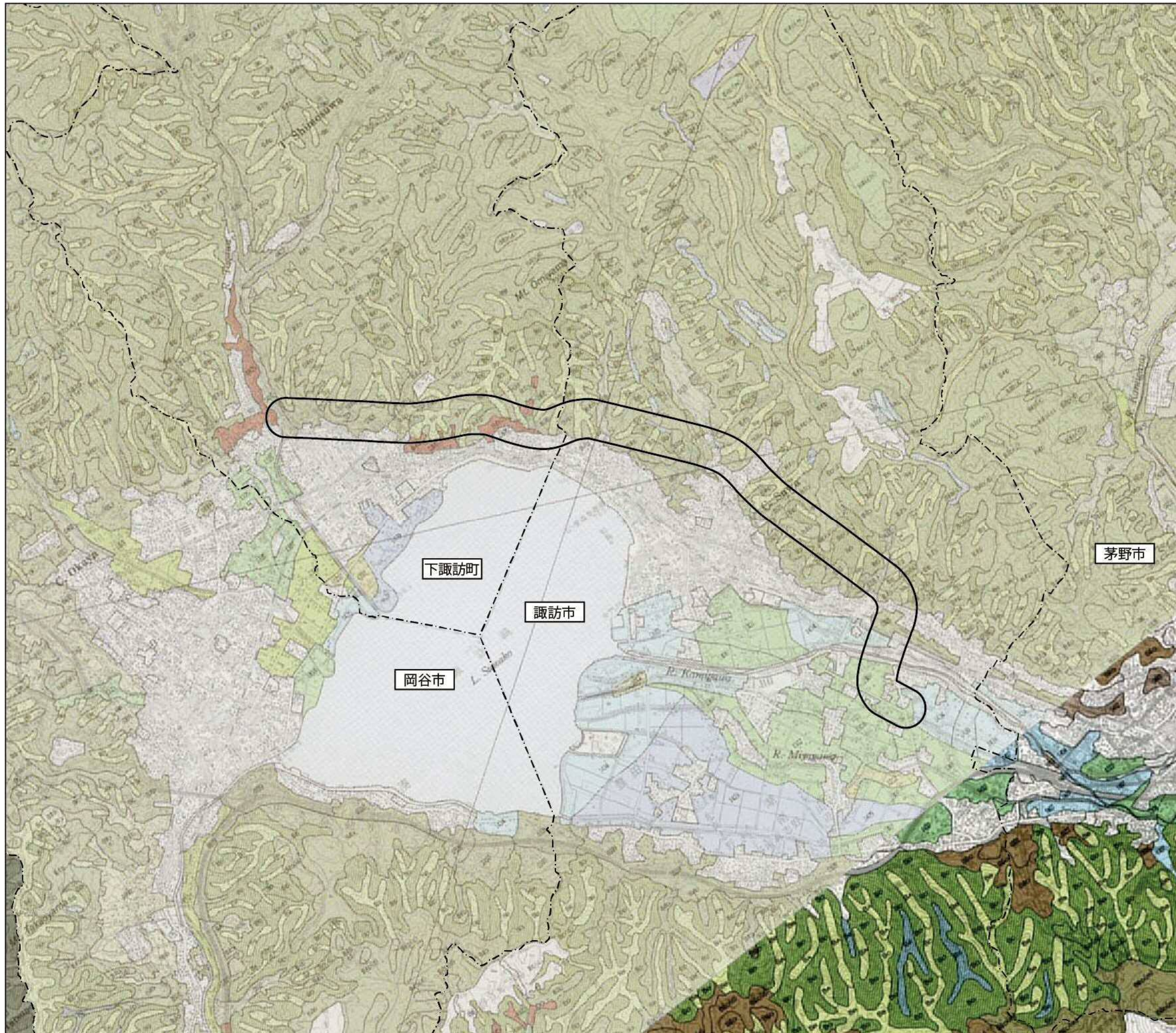
図 4.1.3.1 土壤図
