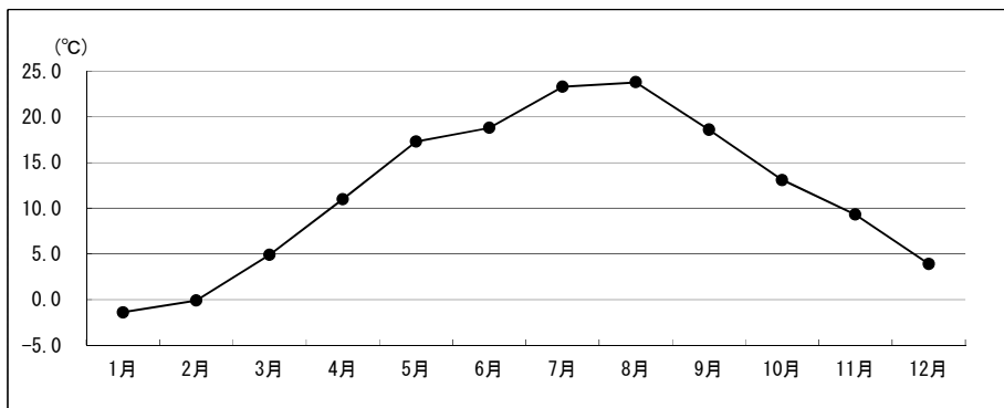
図 4.1.1.2 月平均気温（平成27年）
