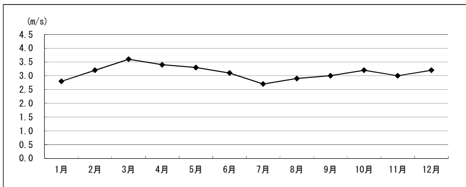
図 4.1.1.4 月別平均風速（平成27年）
