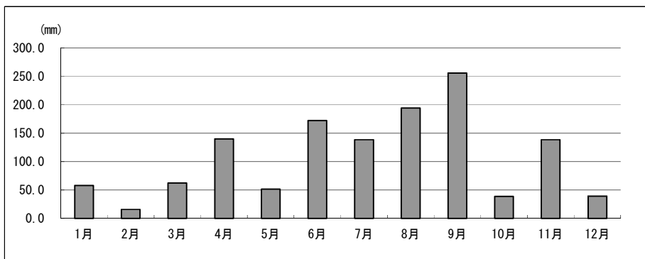
図 4.1.1.3 月降水量（平成27年）
