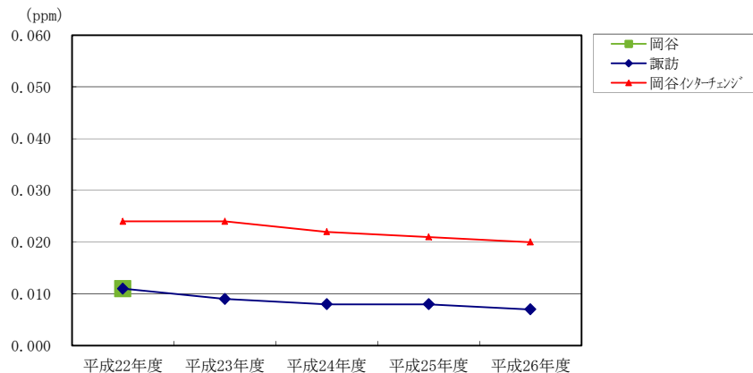
図 4.1.1.7 二酸化窒素 (NO 2 ) の年平均値の経年変化
