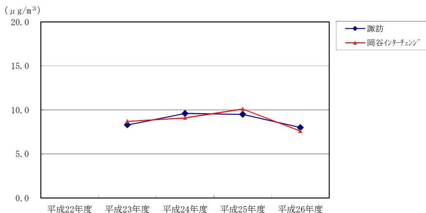
図 4.1.1.10 微小粒子状物質 (PM2.5) の年平均値の経年変化
