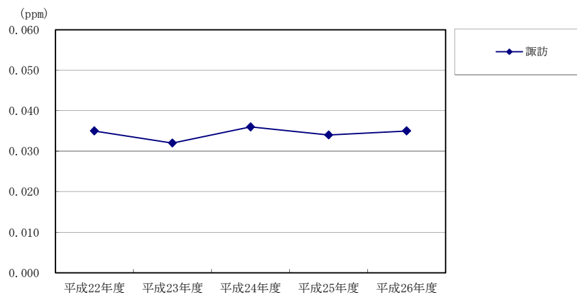
図 4.1.1.9 光化学オキシダント (O x ) の年平均値の経年変化
