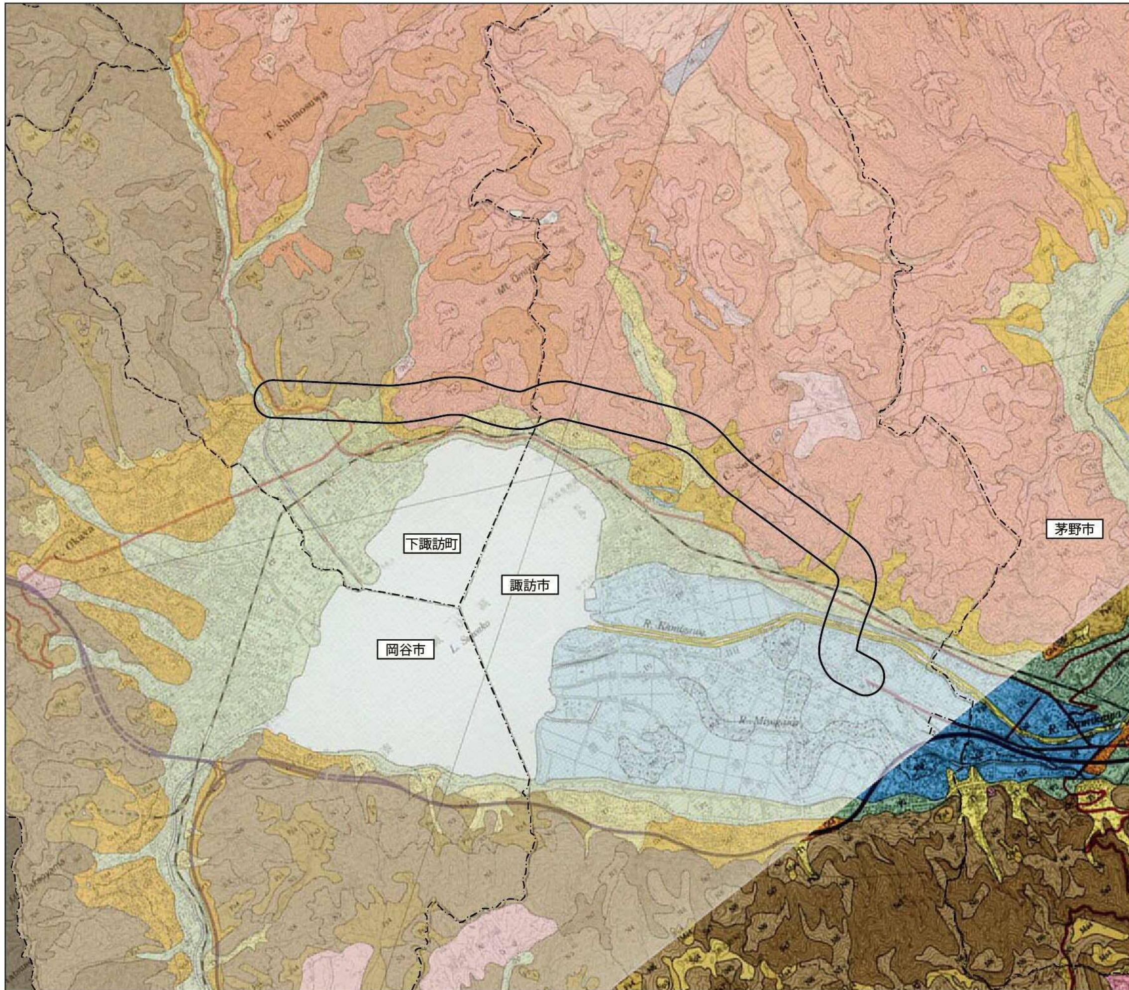
図 4.1.4.1 地形分類図
