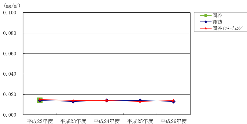
図 4.1.1.8 浮遊粒子状物質 (SPM) の年平均値の経年変化
