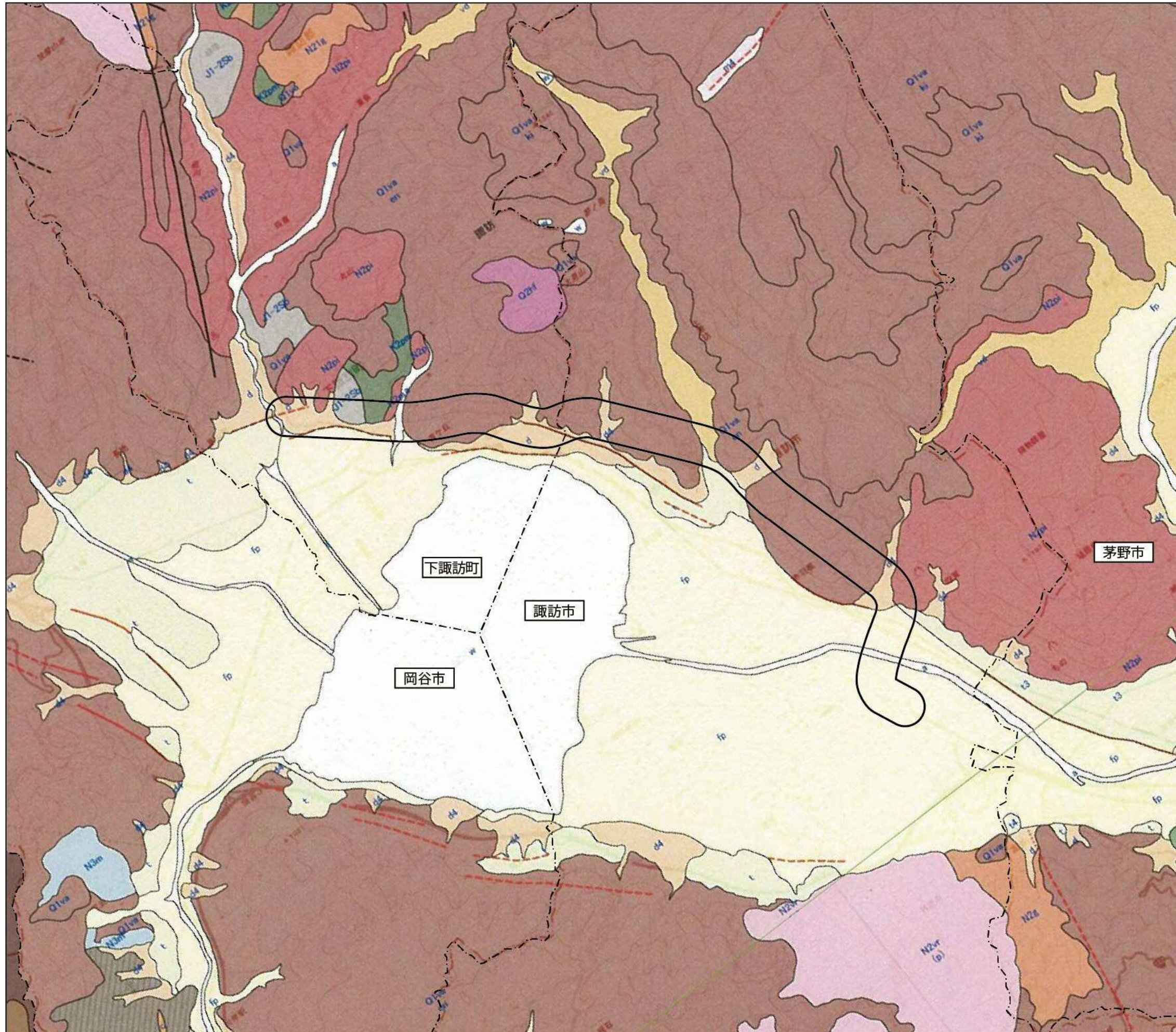
図 4.1.4.2 表層地質図
