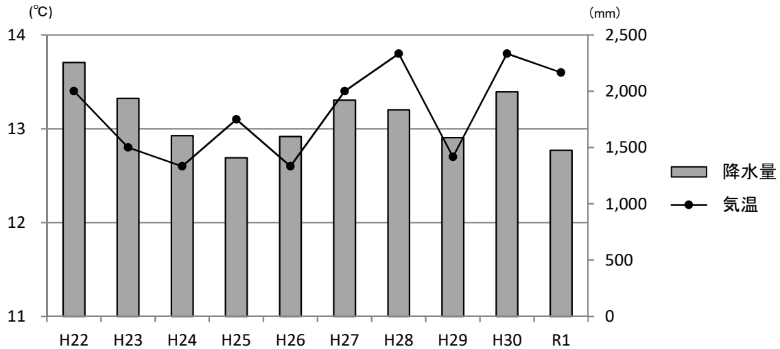
年別平均気温及び降水量の状況
