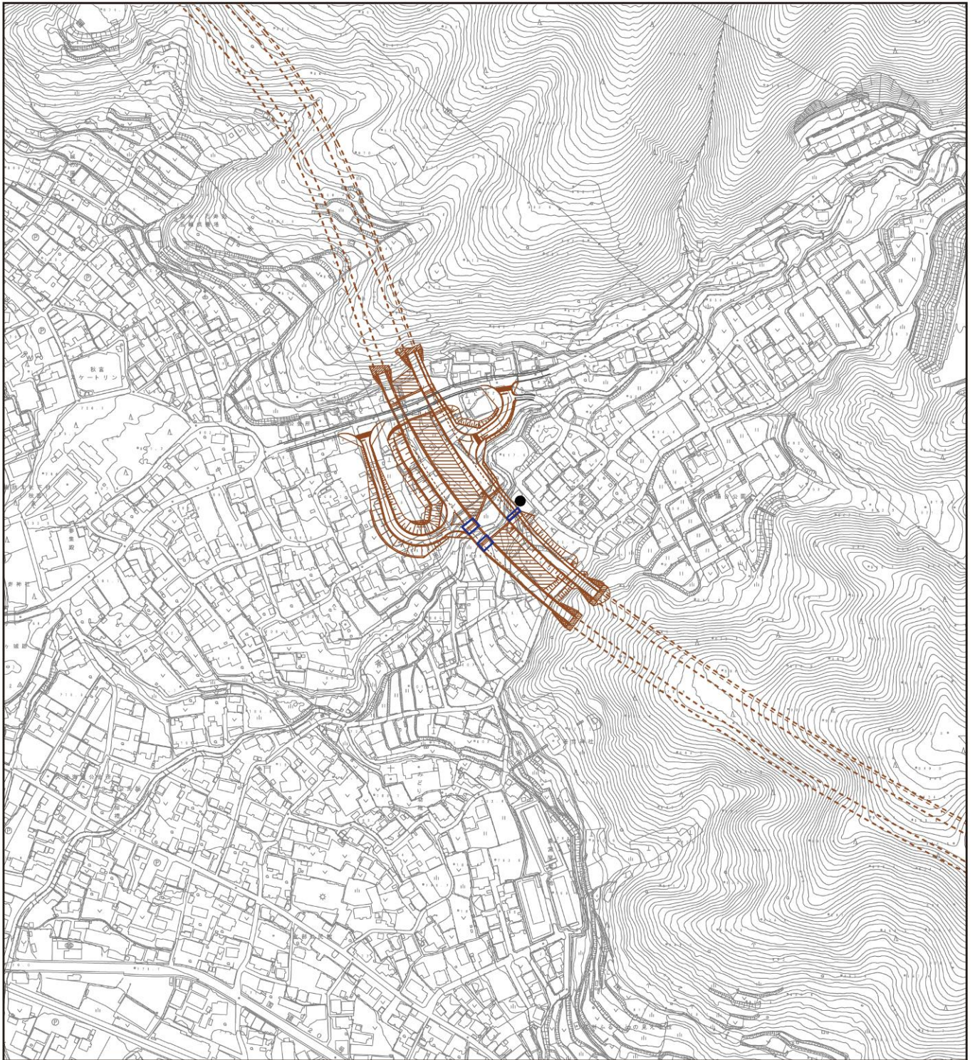
図 2.2.1 (13) 建設機械の稼働に係る粉じん等のユニット配置図 (13. 下諏訪町武居南 2)
