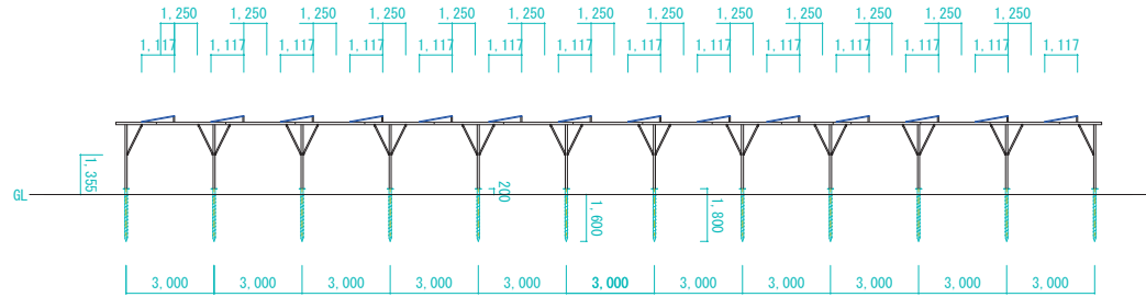
モジュールレイアウト図(1/200)
